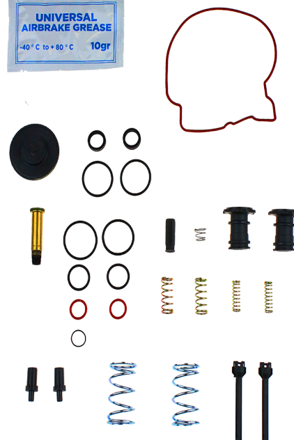
PART No: EKKB.49.5
